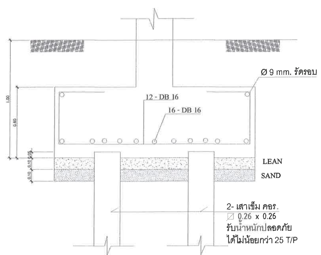
ฐานราก F1 กรณีฐานรากเสาเข็มตอก SCALE 1 : 20
