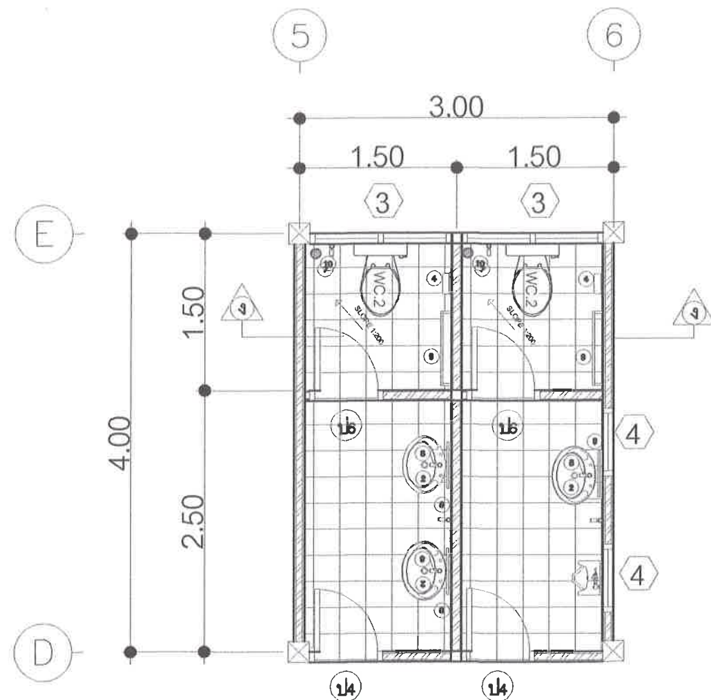
แบบขยายห้อง - น้ำ 1: 25
