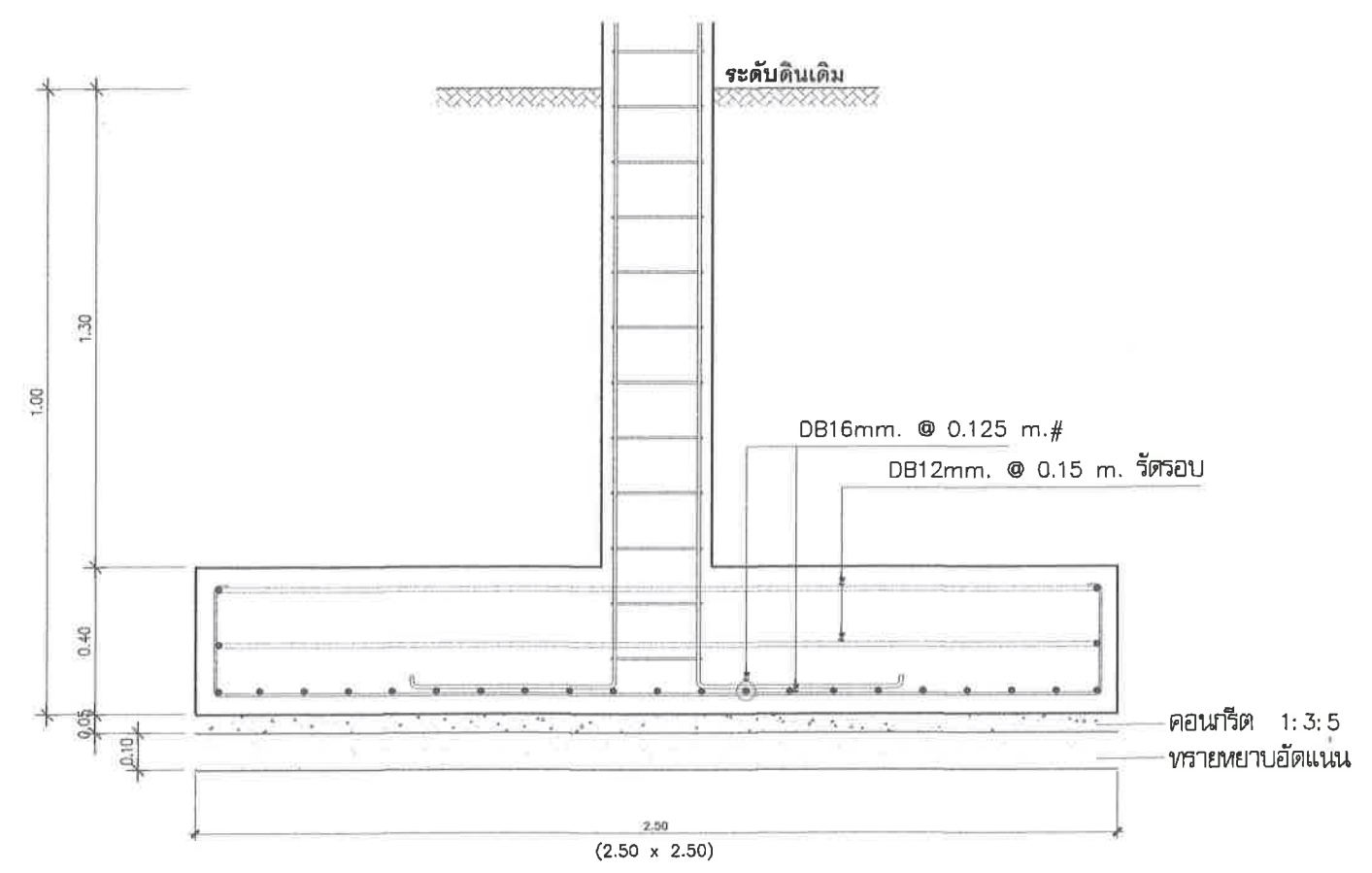
ฐานราก F1 กรณีฐานรากแผ่ ดินรับน้ำหนัก 8 ตัน/ตร.ม. SCALE 1 : 20
