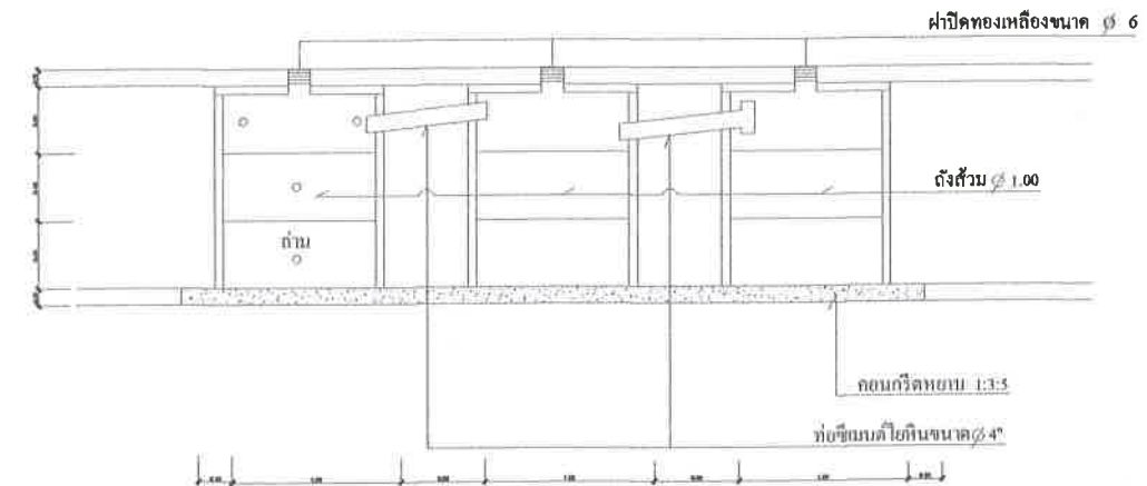
แบบขยายบ่อเกรอะ-บ่อซึม
