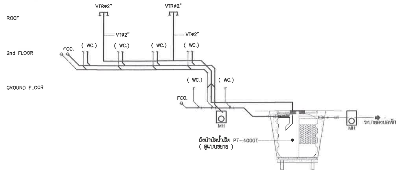
( ตัวอย่าง ) แบบแสดงการระบายน้ำทิ้ง แนวดิ่ง
