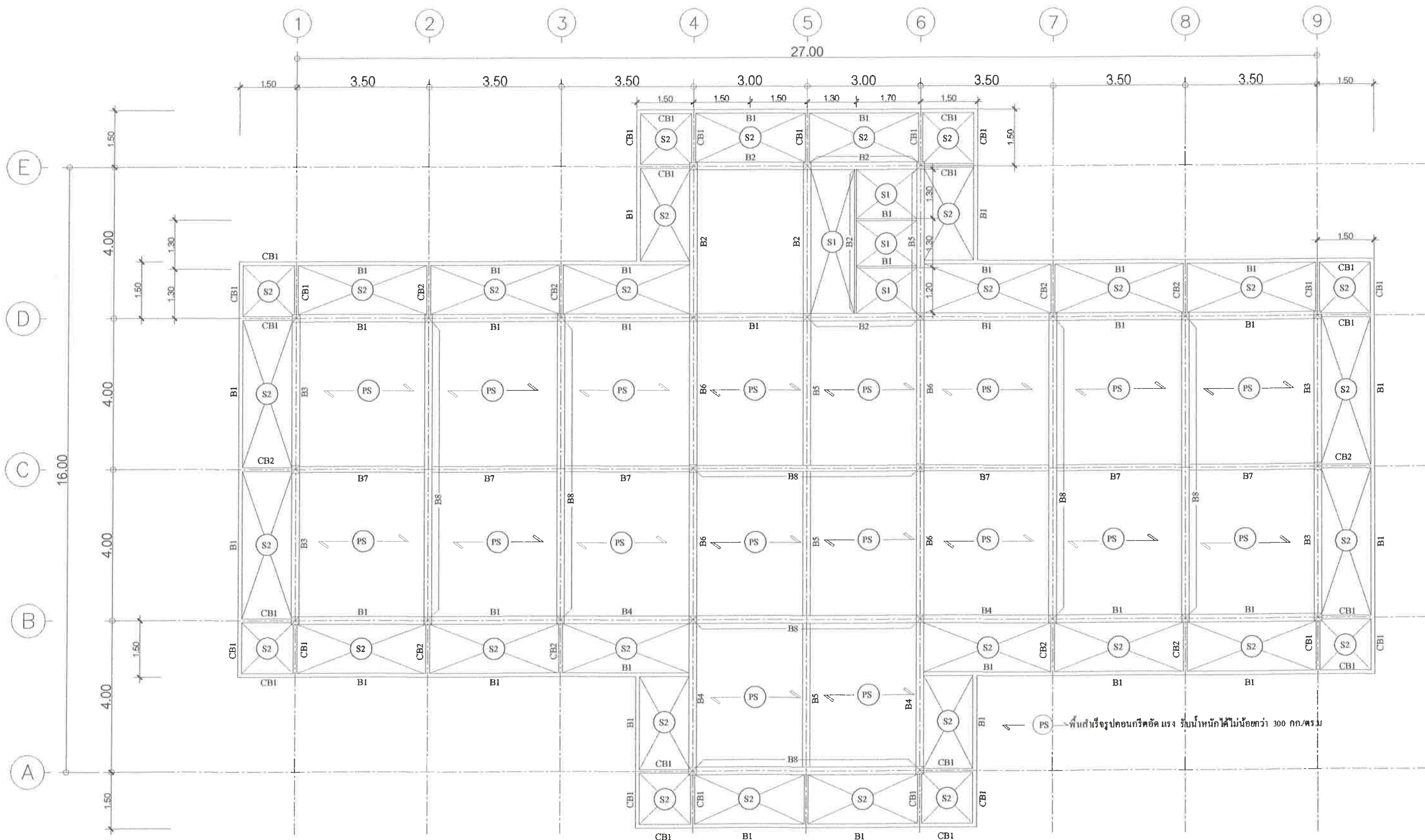
แปลนโครงสร้างพื้นชั้นบน 1 : 100
