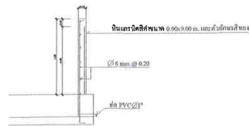
แบบขยายข้อต่อ 1:20
