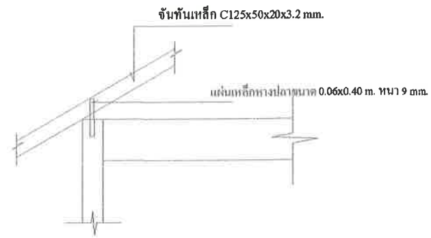
แสดงการยึดจันทันกับเสาหรือคาน คสล.
