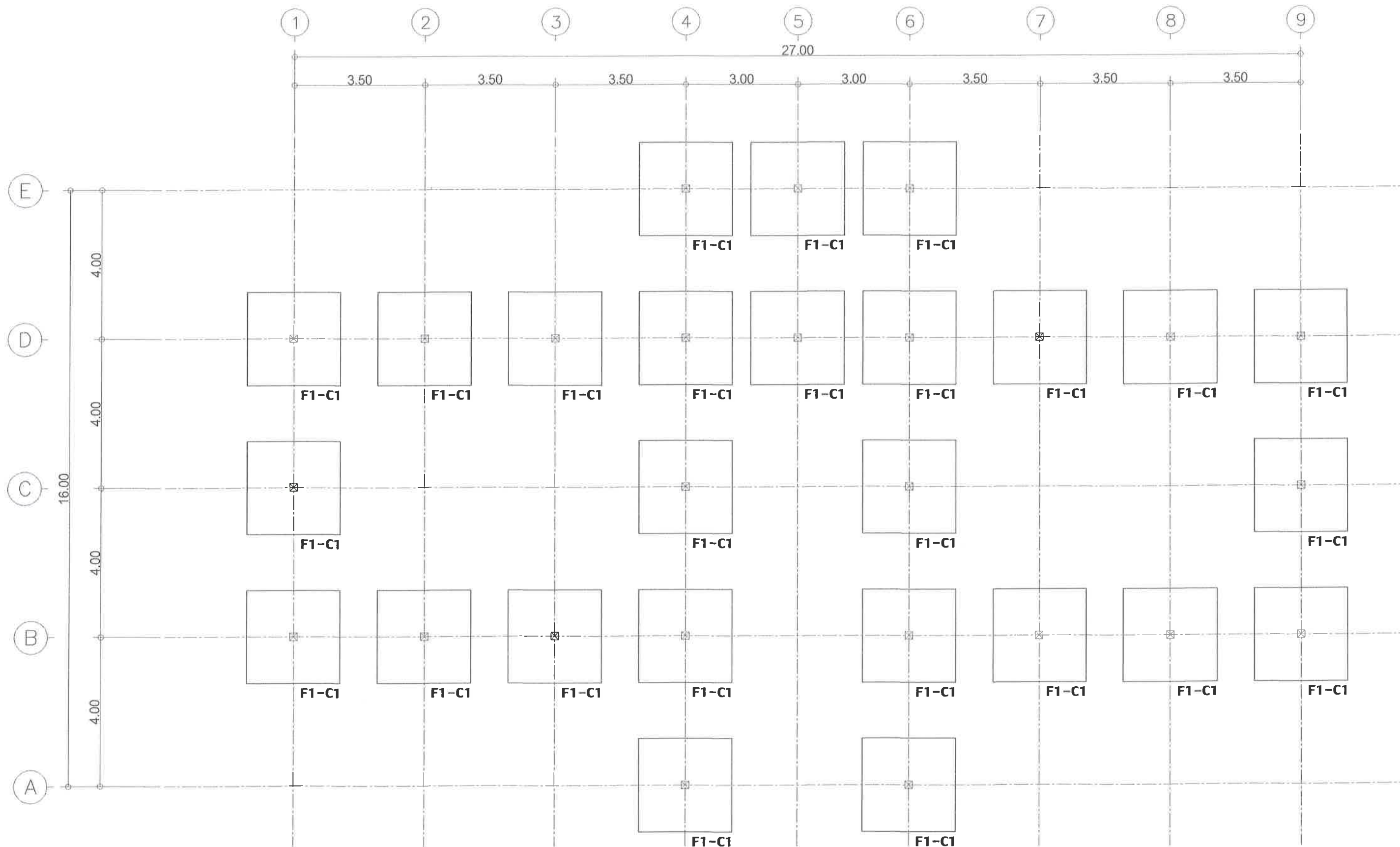
ฐานราก F1 (ฐานรากเพ้) กรณีดินรับน้ำหนัก 8 ตัน/ตร.ม. 1 : 100
