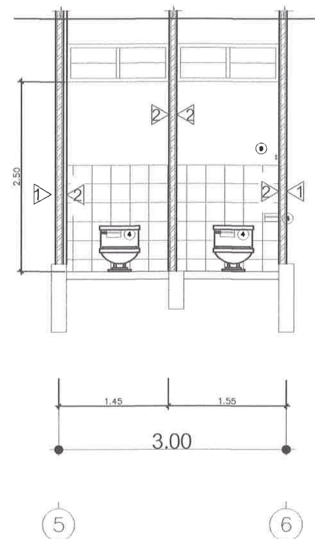
รูปตัดขยายห้องน้ำ-ส้วม ง-ง 1:25
